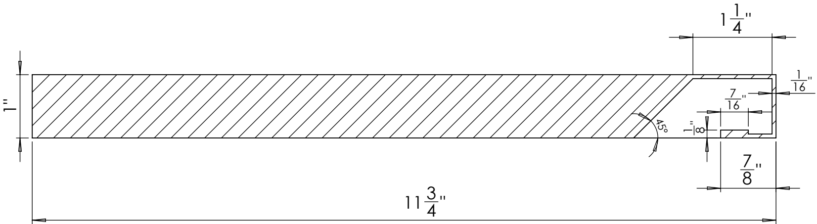
SECTION A-A SCALE 1 : 1.5
